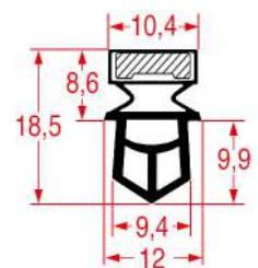
REPA DE PROFILE CODE - 9325
